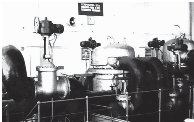
Бойлерная установка
